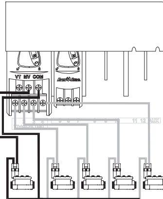
Hauptventil
